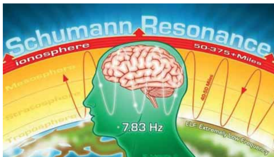
Ionosfera 55 kilometrov nad Zemljo odbija Schumannovo energijo osmih hercev nazaj na Zemljo, od koder se zopet odbije v atmosfero.
